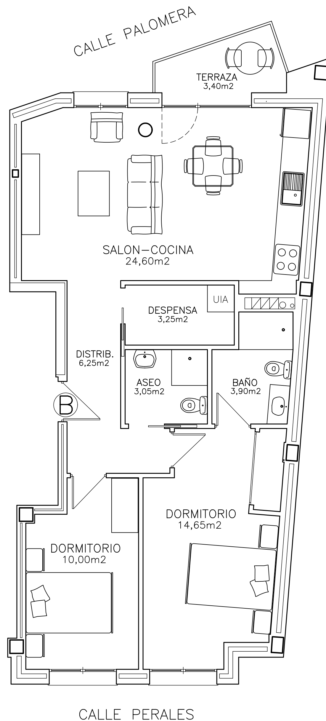
PLANTA TIPO 1ª a 4ª ESC. 1:50 VIVIENDA "B": 65,70m 2 + 3,40m 2 terraza
